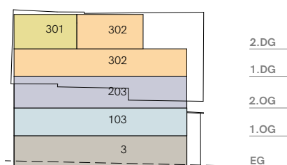
Ansicht West
