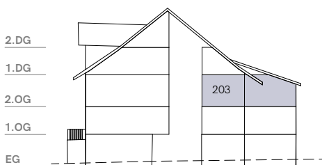
Ansicht Nord
