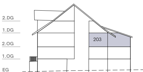
Ansicht Nord
